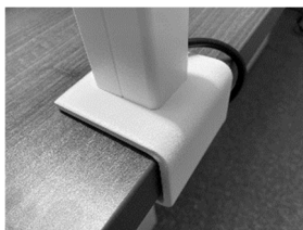
Tischklemme, U-Form abgerundet (Abm. 100x80x60 mm); 230V Kabelauslass seitlich am Standrohr.
